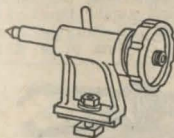
Motdocka № K 604, m. rattmatat, genomborrat dubbör och löstagbar, härdad dubb. Vikt c:a 300 gram. Pris kr. 14:80
