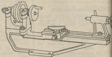
Svarv N:o K 590, med försättare N:o K 606 för handstål samt motdocka med cylindrisk, förskjutbar enkel dubb. Vikt ca 2,2 kg. Pris kr. 36:65
