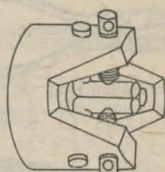
Chuck № K 600, med 3 st. var för sig ställbara, härdade stålbackar. Griper upp till 16 mm. Vikt c:a 200 gram. Pris kr. 12:50
