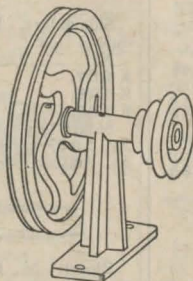
Transmission № K 615 med 150 mm. remskiva samt drivremskiva, lika svarvens. Vikt c:a 1,4 kg. Pris kr. 22:50
