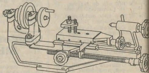
Svarv N:o K 592, lika svarv N:o K 591, men dessutom försedd med ledareskruv N:o K 611. Vikt ca 3,2 kg. Pris kr. 62:50
