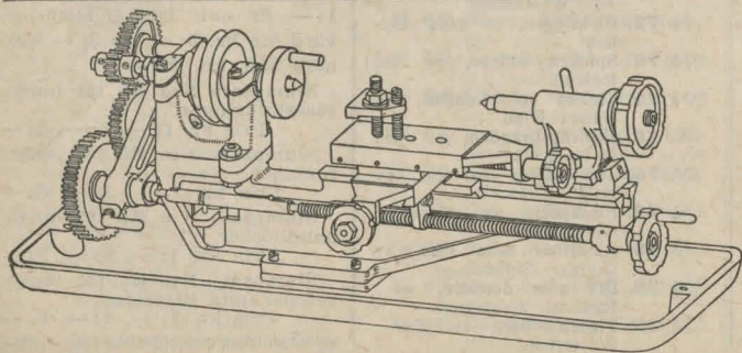
Svarv N:o K 592, lika svarv N:o K 591, men dessutom försedd med ledareskruv N:o K 611. Vikt ca 3,2 kg. Pris kr. 62:50
