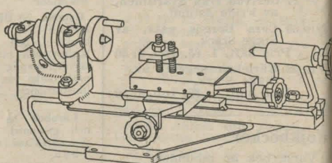
Svarv N:o K 591, lika svarv N:o K 590, men med korsupport N:o K 610 i stället för försättare. Vikt ca 3 kg. Pris kr. 52:70
