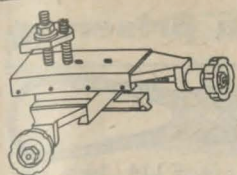
Korsstöd № K 610. Vikt c:a 860 gram. Pris kr. 22:—
