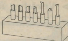
Svarvstålsats № K 616, med 7 st. olika svarvstål. Runda 5 mm. av kolstål, härdade och anlöpta. I träklot. Vikt c:a 35 gr. Pris kr. 5:60
