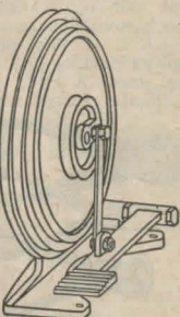
Fotdrift № K 613, med 3 st. hastigheter och en liten extra remskiva för låga varvtal och stor dragkraft. Diam. 300 mm. Vikt c:a 11 kg. Pris kr. 39:50 Svånghjul № K 614, m. vevstake och pedal. Lika № K 613, men för montage i bänk. Utan ställ. Vikt c:a 8 kg. Pris kr. 33:75
