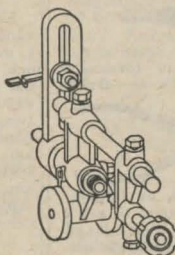
Delningsapparat № K 594, fästes på vertikalsliden eller på verktygssliden i vinkelhylla. Spindelnsen lika svarvens. Svarvens växelhjul användas för delning Kombinerad delning möjlig. Användes vid fräsning av kugghjul, gradering m. m. Utan kugghjul. Vikt c:a 800 gr. Pris kr. 39:50
