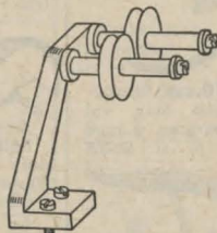
Remledarearm № K 595, med två bryttrullar. Att användas vid drift under bänk av svarv med automatisk matning, med eller utan oljetallrik. Vikt c:a 500 gram. Pris kr. 12:85
