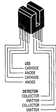
CASE 792-01
