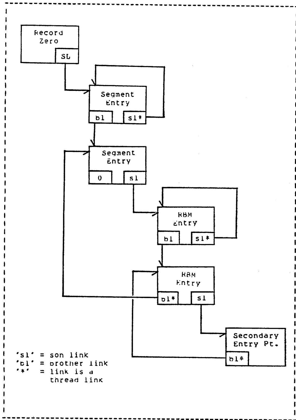
Illustration 3.4.1.3 -- Segment List
