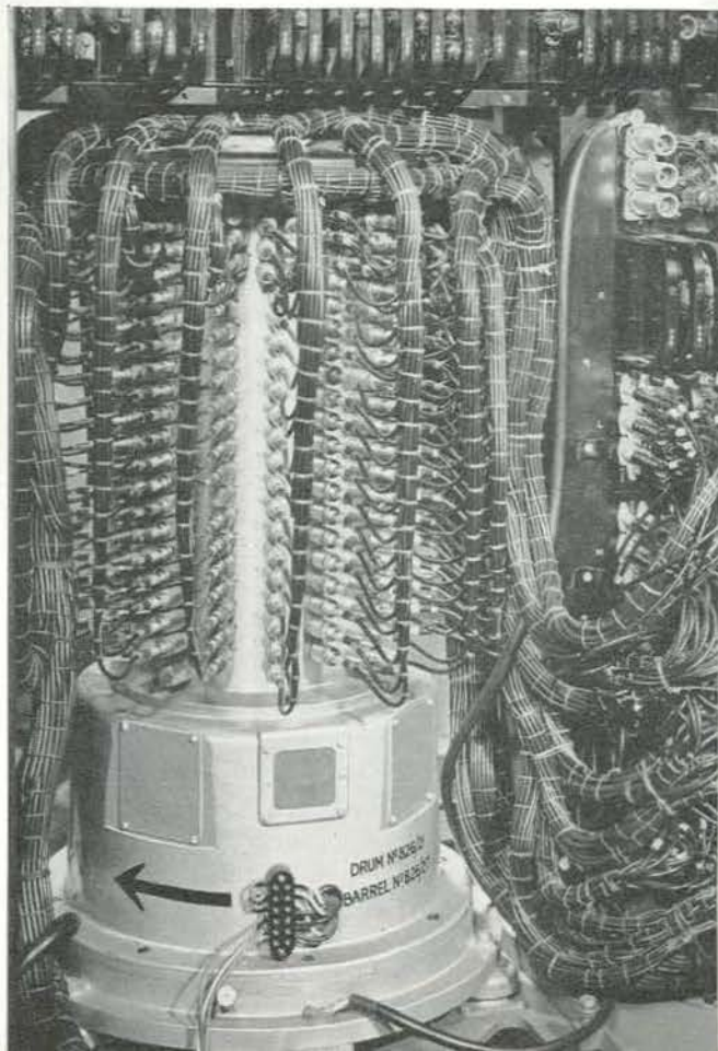
STANTEC-ZEBRA Main Store.
