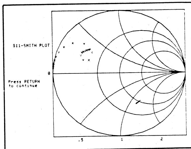
Fig. 11. Input S-parameter.
